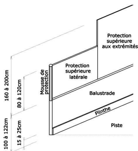
Détail balustrade
